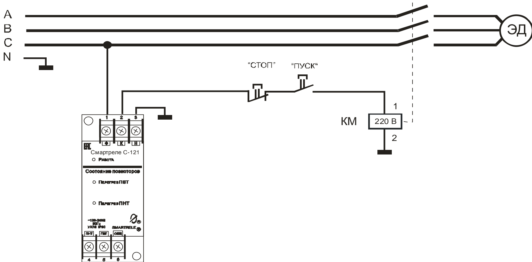
Рисунок 3 – схема включения реле в систему управления электродвигателем
